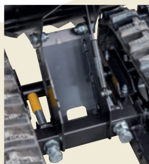
Ribaltamento manuale con pistone a gas
